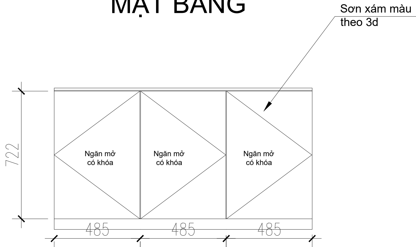
MẶT ĐỨNG
