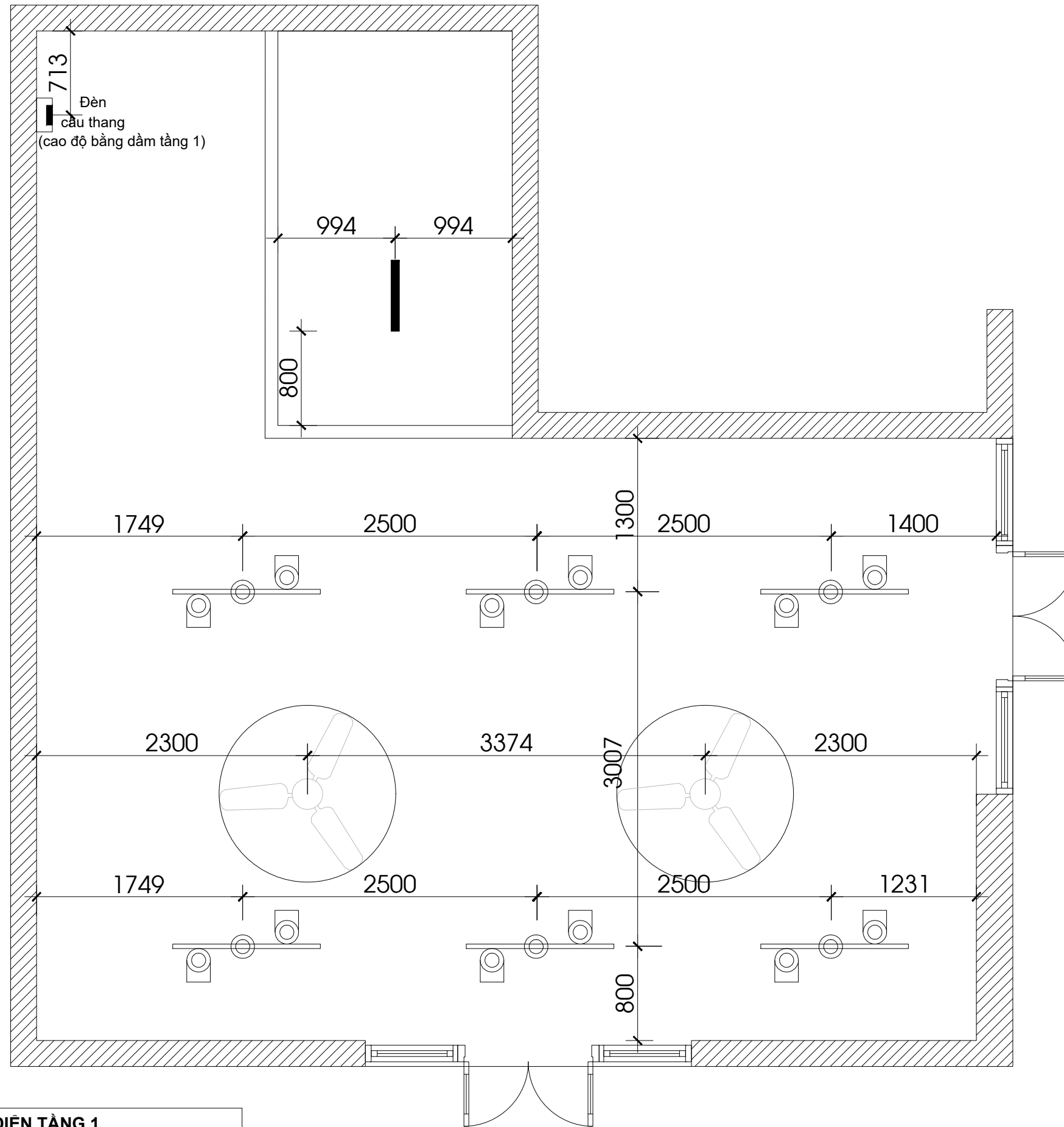
Đèn ray rọi 3 bóng
