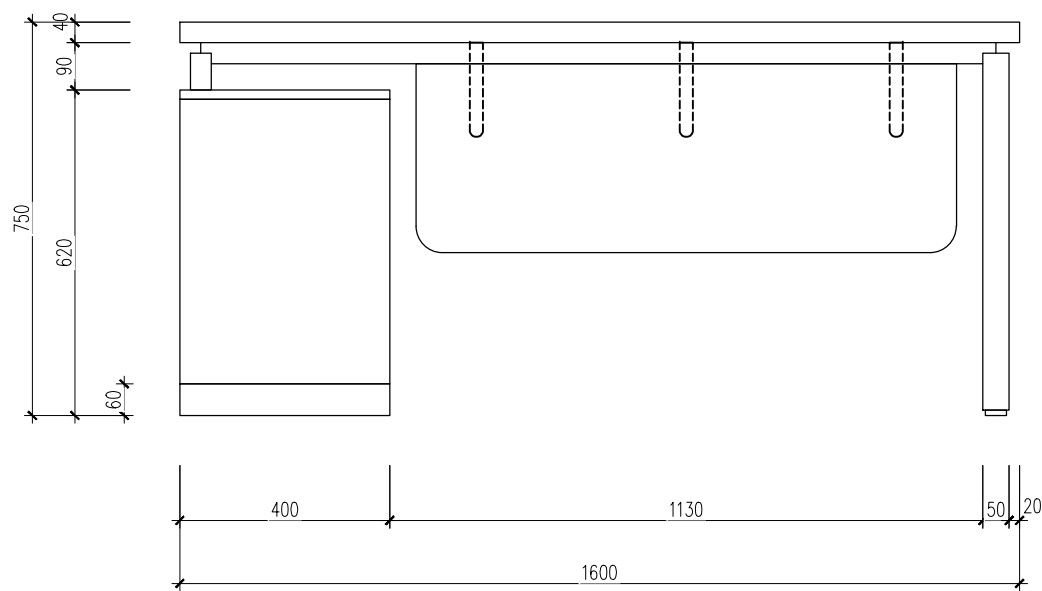
MẶT ĐỨNG
