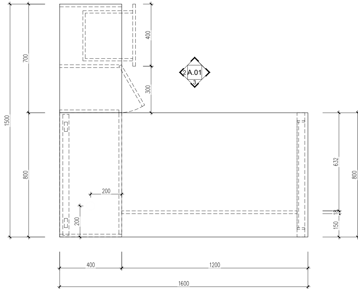
MẶT BẰNG
