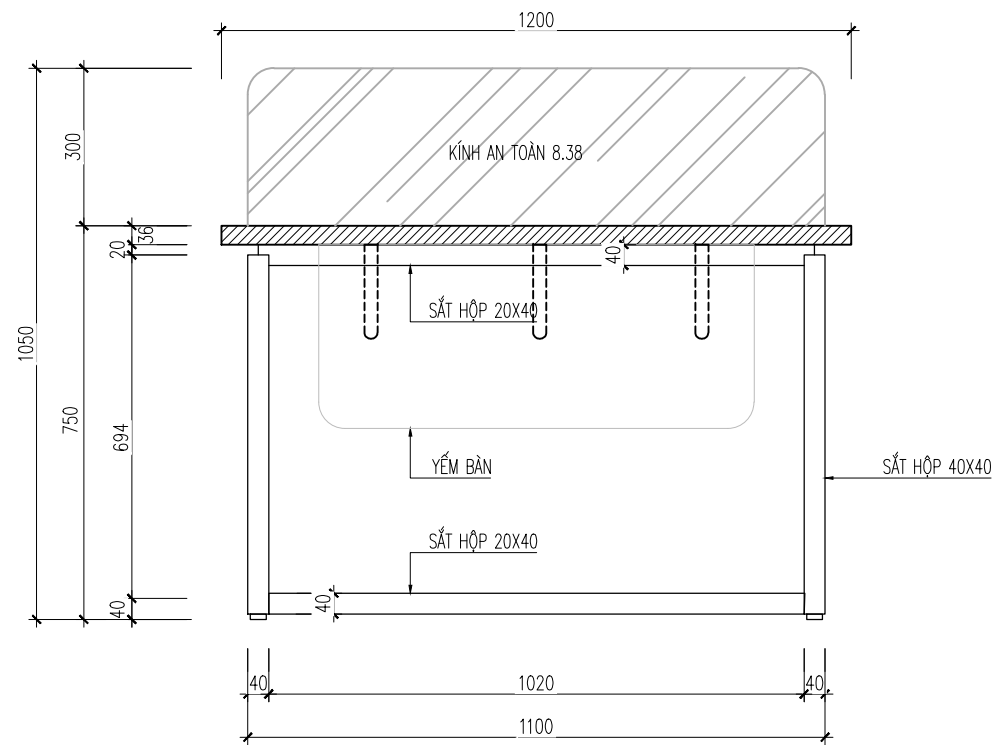
MẶT ĐÚNG
