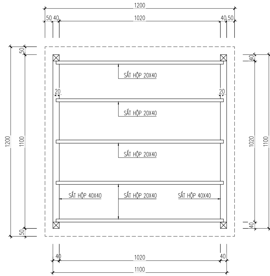
CHI TIẾT CHÂN SẮT
