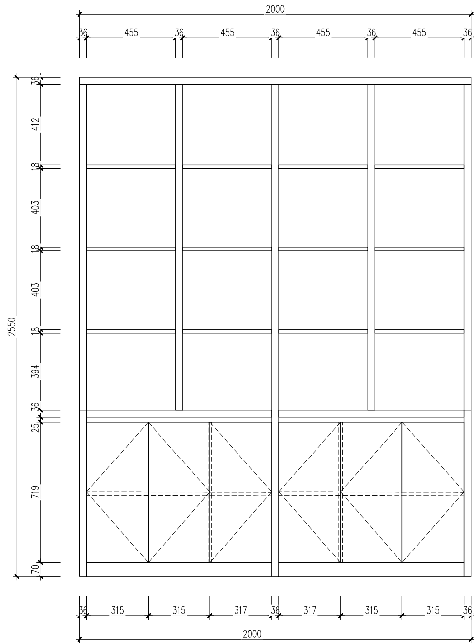
MẶT ĐÚNG
