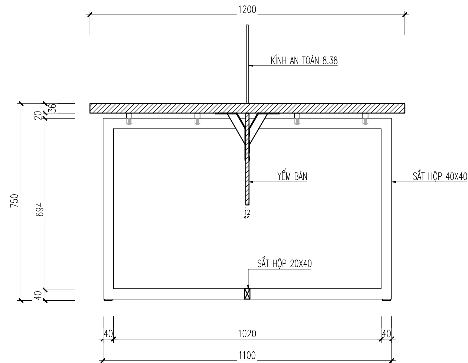
MẶT BÊN
